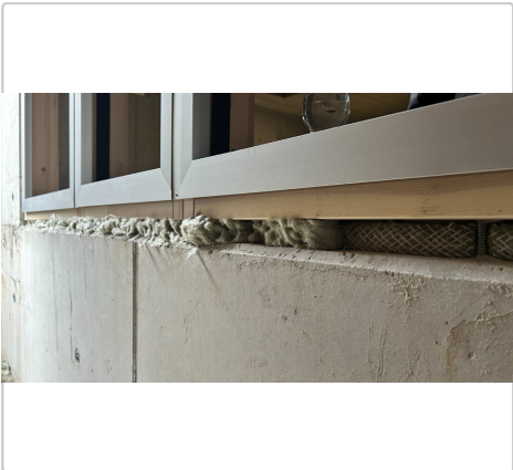
Vykonaná práca 3: Lepenie namontovaných fasád na športovej hale pre hornú PR fasádu, pohľad juh A22 02. 06. 2026 21:52
