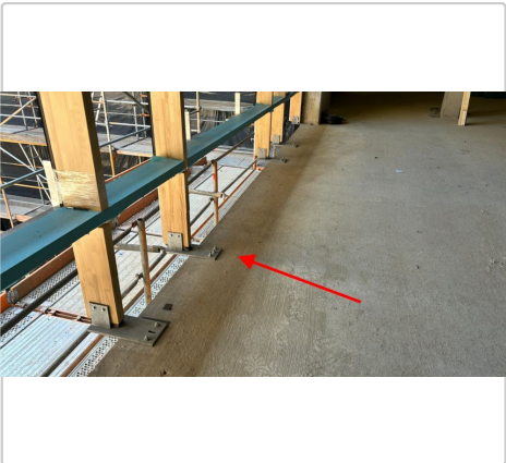
Uitgevoerde werk 1: Montage van de onderste consoles voor de PR-gevel bij de sporthal, zuidzijde, A25–A27 26-06-2026, 08:35
