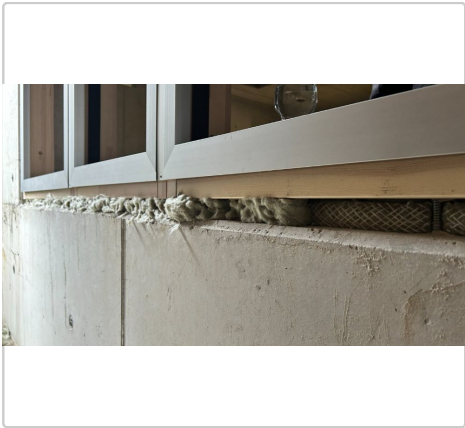
Elvégzett munka 3: A felszerelt homlokzatok ragasztása a sportcsarnoknál a felső PR homlokzathoz, déli nézet A22 2026. 06. 02. 21:52
