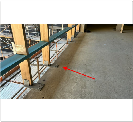
Elvégzett munka 1: Az alsó konzolok szerelése a PR homlokzathoz a sportcsarnoknál, déli nézet, A25–A27 2026. 06. 26. 08:35
