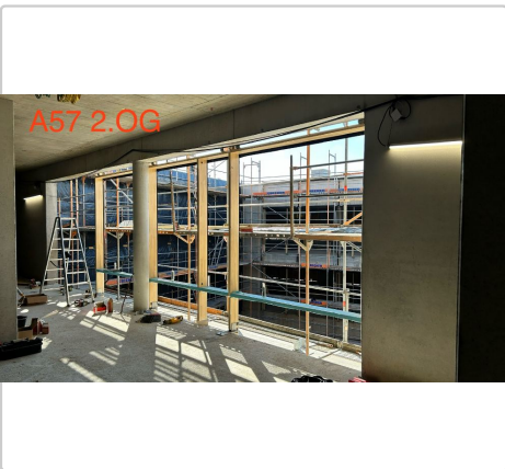
Travail exécuté 4 : Alignement des éléments de façade et montage des consoles supérieures pour la façade PR au gymnase, vue ouest, A24 25/06/2026 09:49
