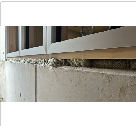
Travail exécuté 3 : Collage des façades montées au gymnase pour la façade PR supérieure, vue sud A22 02/06/2026 21:52
