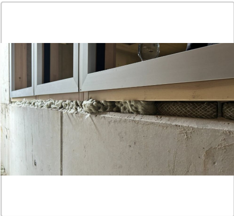
Trabajo realizado 3: Pegado de las fachadas montadas en el polideportivo para la fachada PR superior, vista sur A22 02/06/2026, 21:52
