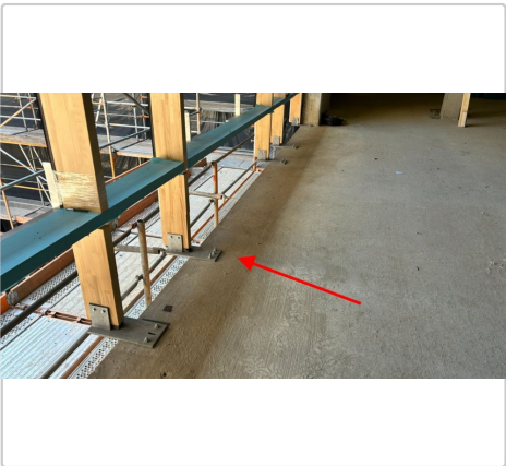
Trabajo realizado 1: Montaje de los soportes inferiores para la fachada PR en el polideportivo, vista sur, A25–A27 26/06/2026, 08:35
