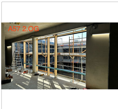
Ausgeführte Arbeit 4: Ausrichten der Fassadenelemente und Montage der oberen Konsolen für die PR-Fassade an der Sporthalle, Ansicht West, A24 25.06.2026, 09:49
